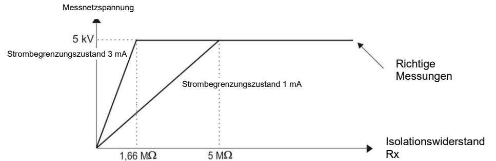
Die eigentliche Messspannung in der Funktion des gemessenen Isolationswiderstandes Rx (für die maximale Messspannung)
